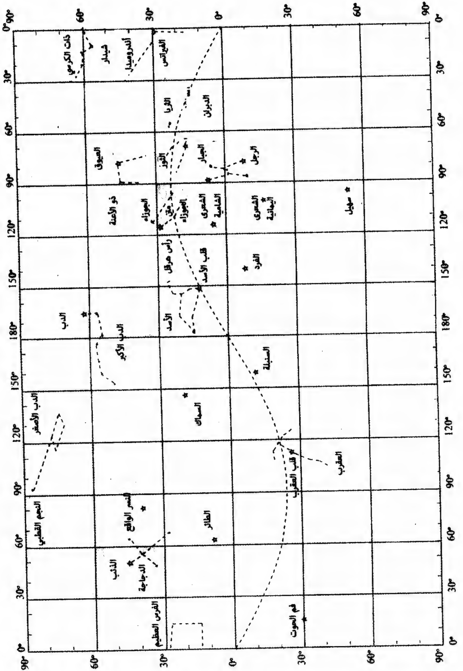
الشكل (59): خارطة سماوية لنجوم الملاحظة الرئيسة. اميل ممثل على المحور العمودي، وخط الطول السماوي مرسوم ليتعلق بخط الطول الأرضي. مسار الشمس خلال العام مبين على شكل خط منقط.
